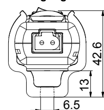
Schraubbefestigung M6
